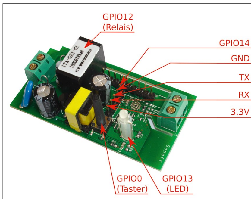
Abbildung 3: Ein um eine Stiftleiste erweitertes Sonoff-Modul.
