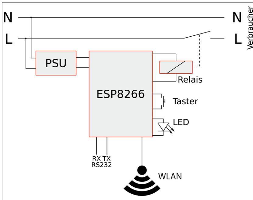
Abbildung 2: Blockschaltbild des Sonoff-Moduls.
