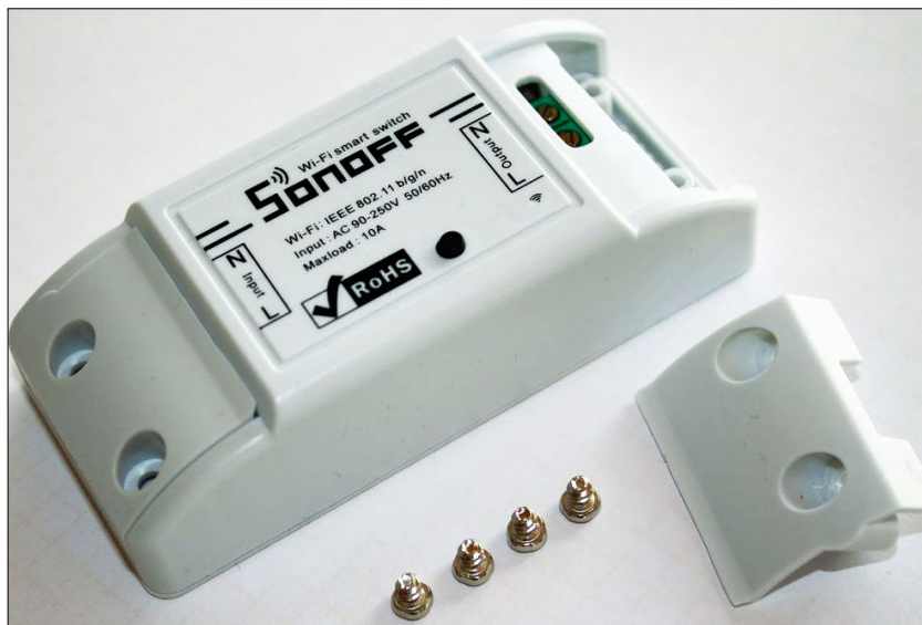
Abbildung 1: Lieferumfang eines Standard-Sonoff-Moduls.
